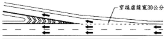
單車道直接式出口
