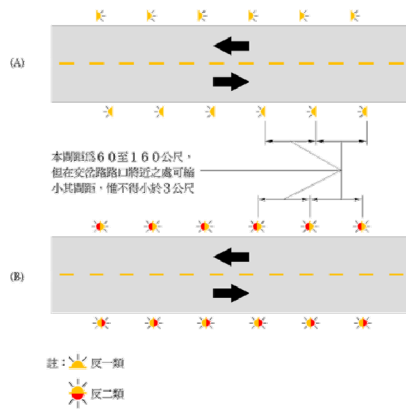
圖一 公路直線上反光導標之位置
