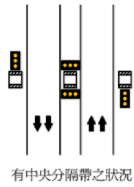
圖七 多車道上危險標記之設置
