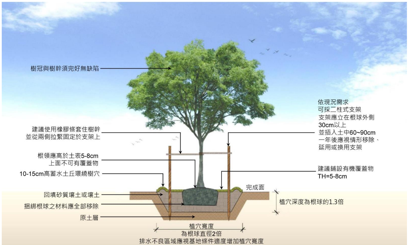
樹木種植與支架詳圖 (二支柱)
