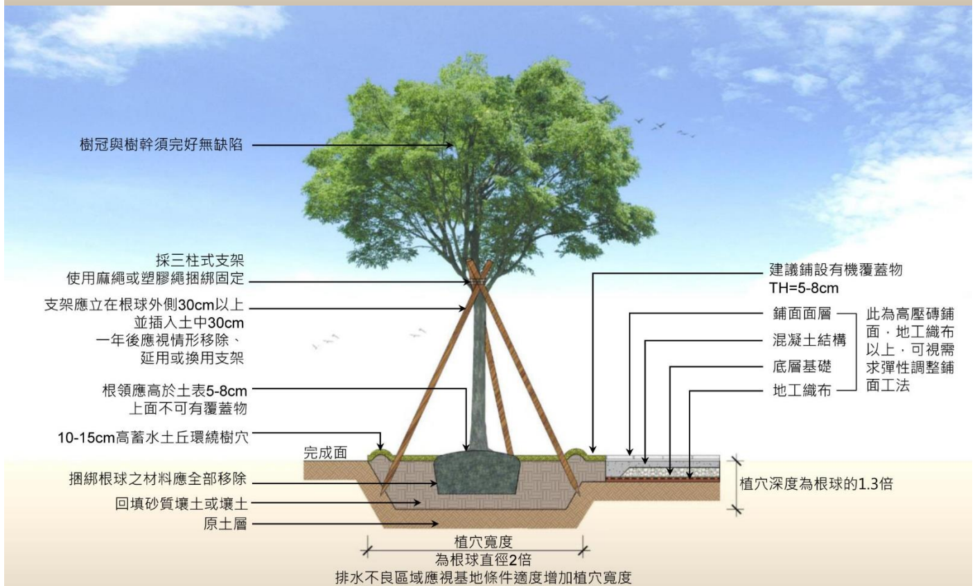
樹木種植與支架詳圖 (三支柱)
