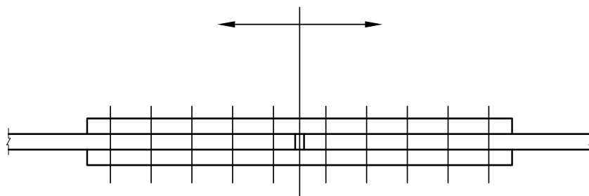
圖 05121-1 栓緊順序
