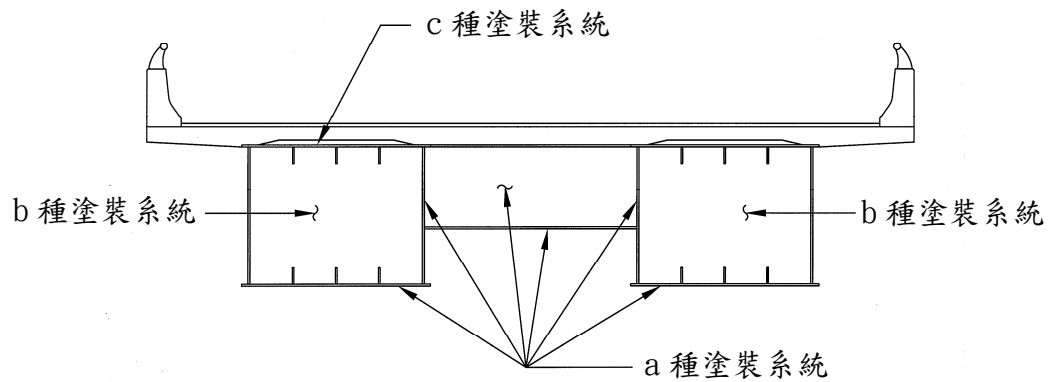
圖 09972-2 鋼箱型梁橋塗裝示意
