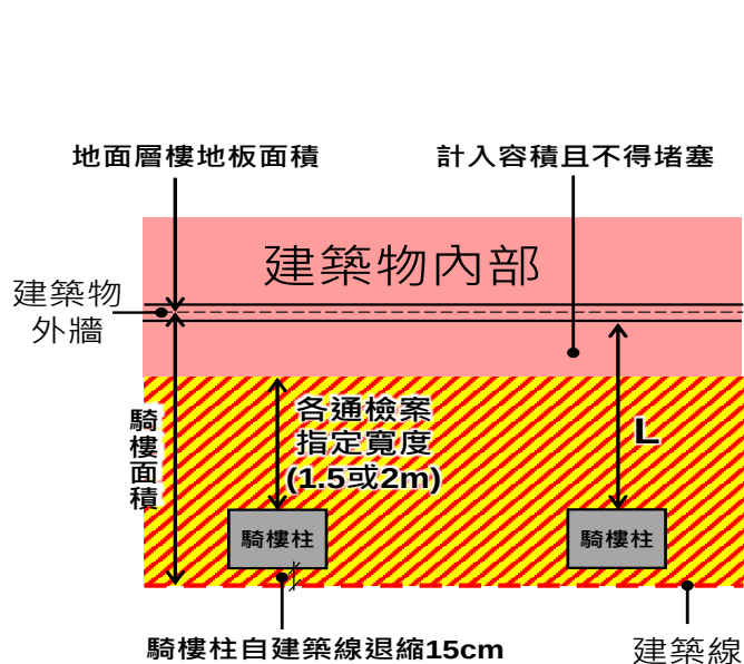
平面圖
