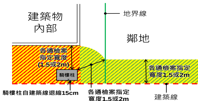
平面圖
