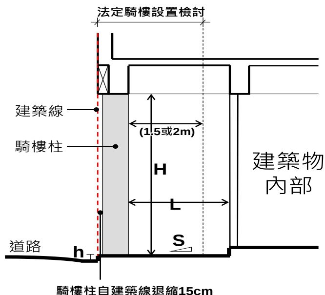
剖面圖
