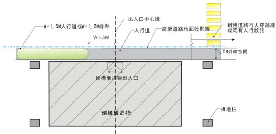
附圖五: 構造物出入口位於車道側時， 人行道留設方式示意圖
