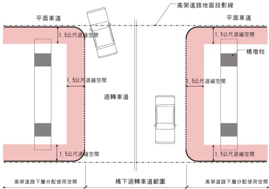
附圖三:1.5公尺退縮空間平面示意圖 (橋下迴轉車道邊線退縮)
