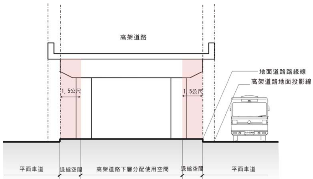
附圖二:1.5公尺退縮空間剖面示意圖 (地面道路路緣線在高架道路地面投影線之內)
