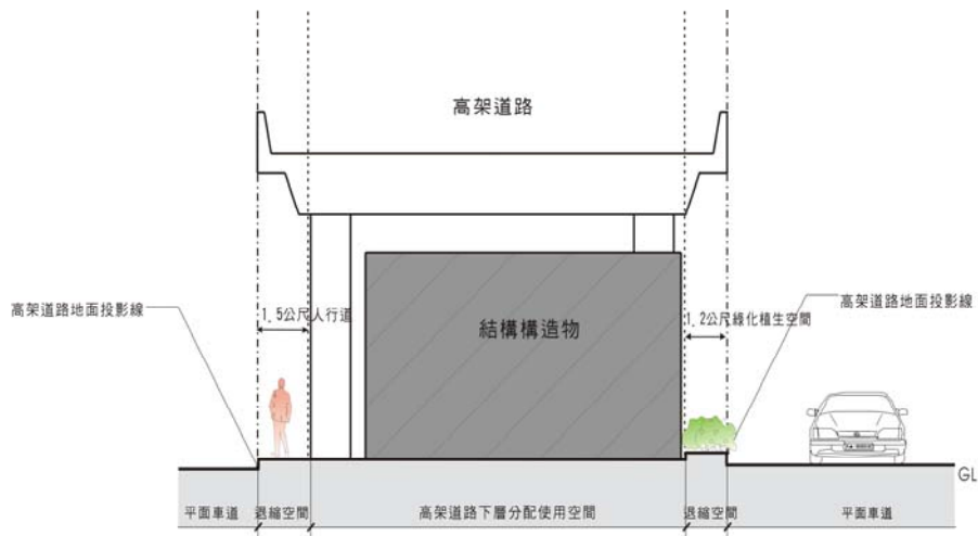
附圖四:高架道路下層構造物退縮1.5公尺人行道 或1.2公尺綠化植生空間剖面示意圖
