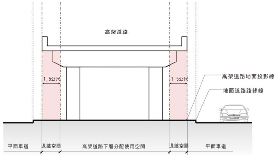
附圖一:1.5公尺退縮空間剖面示意圖 (地面道路路緣線在高架道路地面投影線之外)
