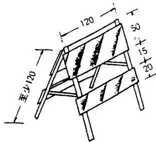
金屬或其他材料活動型拒馬 (單位：公分)
