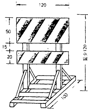
木質活動型拒馬 (單位：公分)
