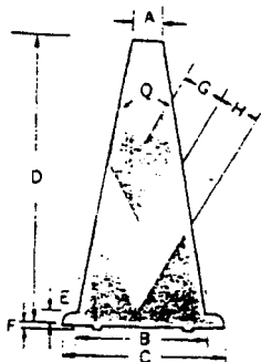
圖一 交通錐 單位：公分
