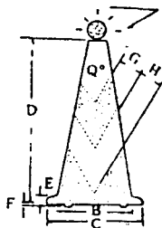
圖二 交通錐加裝警示燈
