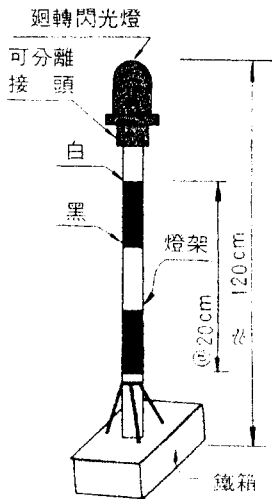
直流式附電瓶警告燈號
