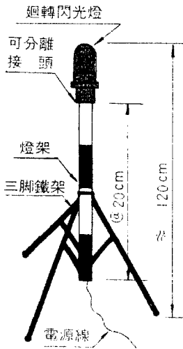
交流式附三腳架警告燈號
