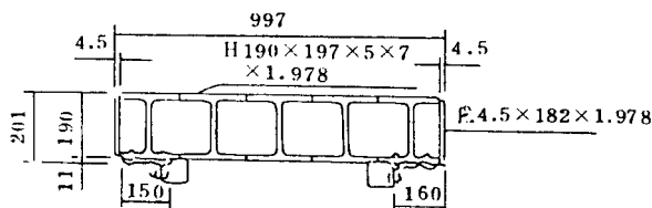
圖三之一 H型鋼覆盖板斷面圖
