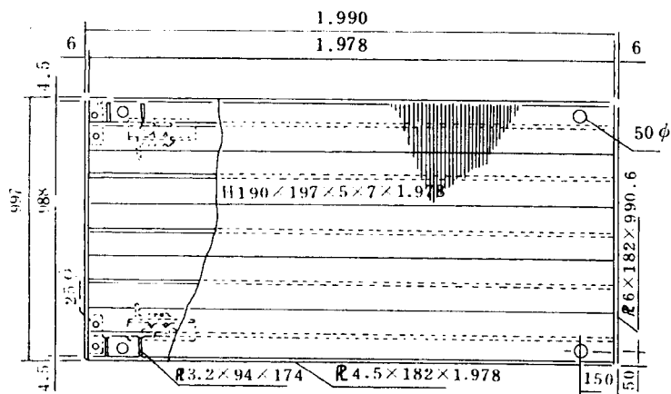
圖三之一 H型鋼覆盖板平面圖
