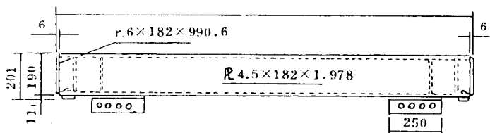
圖三之一 H型鋼覆盖板側面圖
