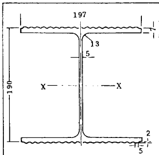
圖三之一 H型鋼断面尺寸
