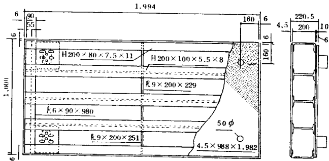
圖三之二 H型鋼覆蓋板組之圖
