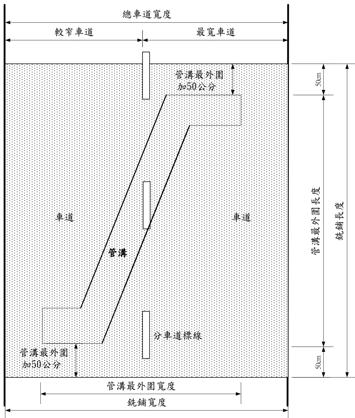
附圖二 瀝青混凝土銑鋪路面修復範圍圖(示意圖) (管溝位於2車道或以上範圍者)
