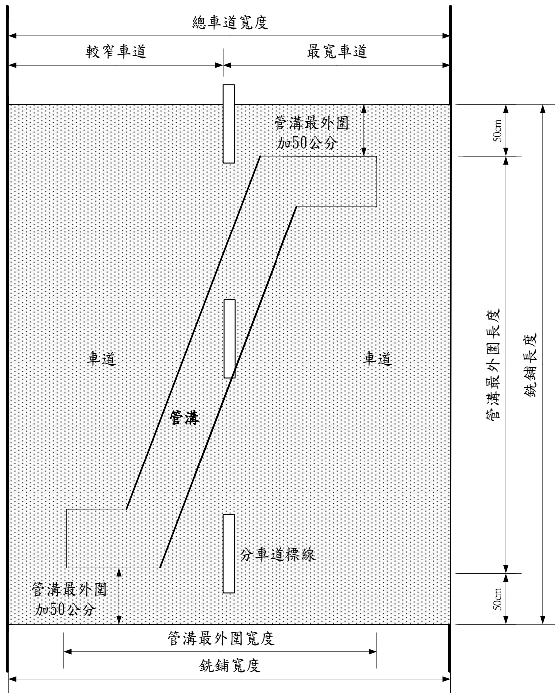
附圖二 瀝青混凝土銑鋪路面修復範圍圖(示意圖) (管溝位於2車道或以上範圍者)
