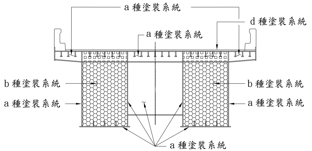
圖 09972-1 鋼橋面板橋塗裝示意
