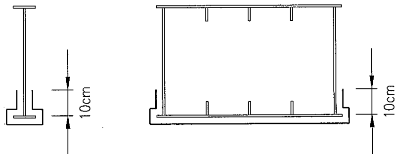
圖 09972-2 鋼箱型梁橋塗裝示意
