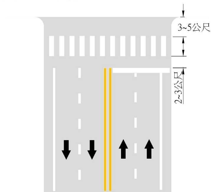
圖一 直交路口
