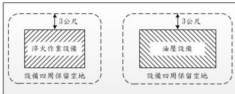
俯視圖
