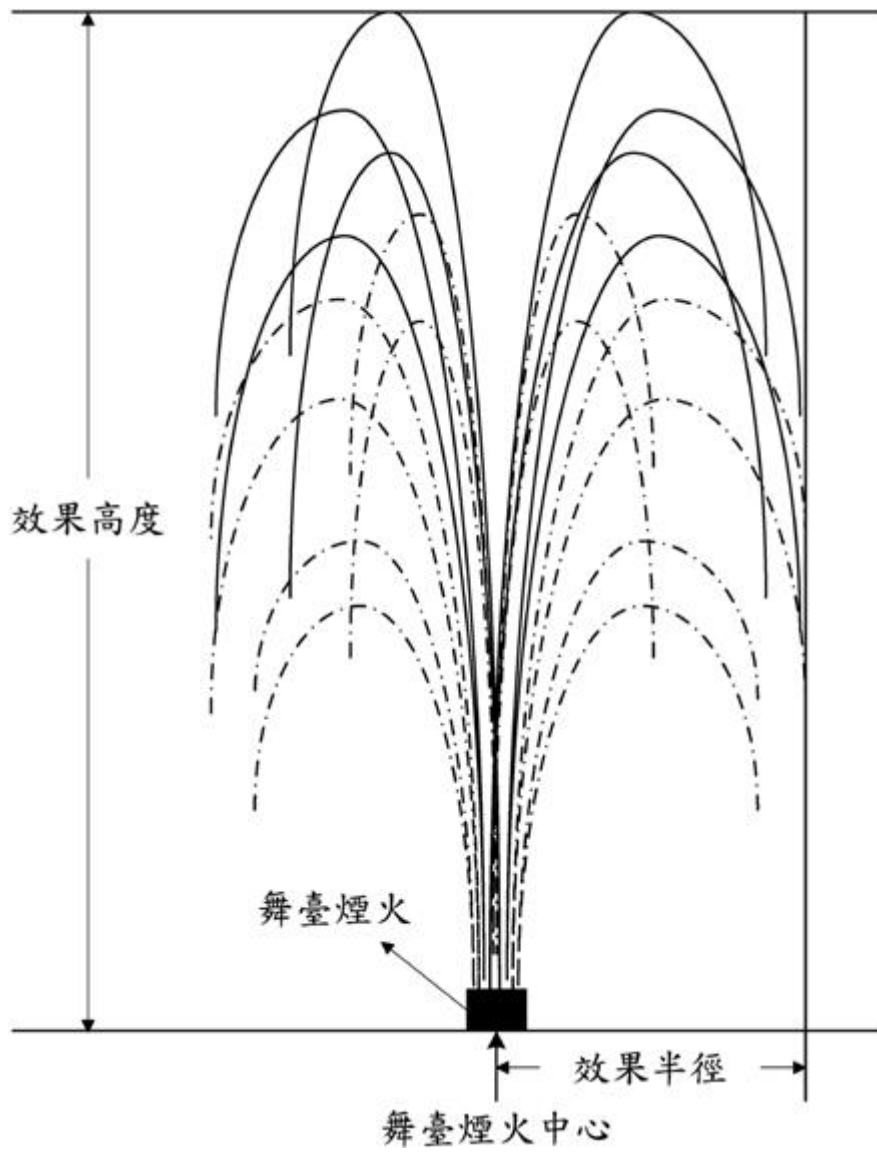
舞臺煙火之效果半徑及效果高度
