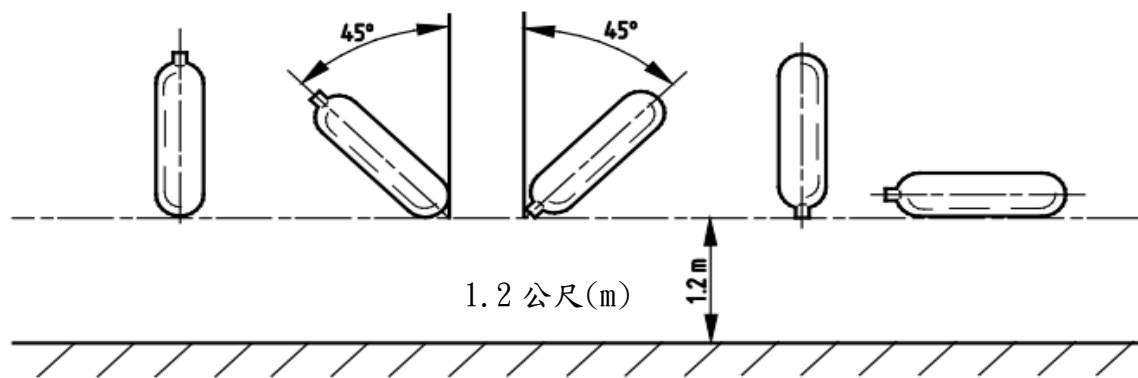
圖十九 摔落試驗
