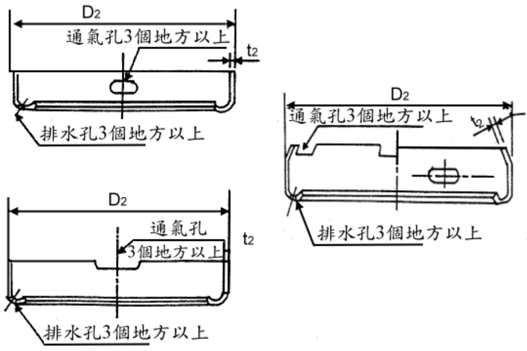
圖六 鋼裙形狀及尺寸
