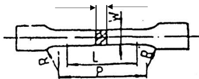
五號試驗片 (CNS2112)
