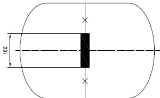
圖十四 焊道照射長度：僅有一條周向接頭之鋼瓶
