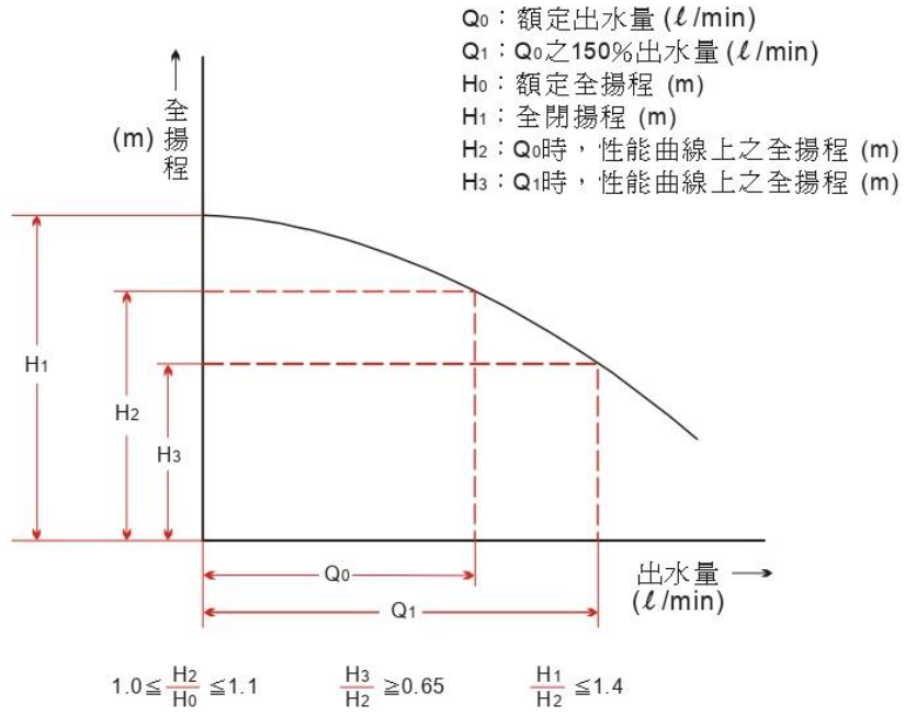
附圖1 性能曲線圖
