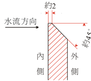
圖1 堰板之截面圖 (單位：mm)
