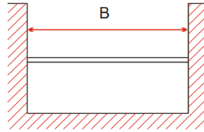
圖5 全幅堰之堰緣
