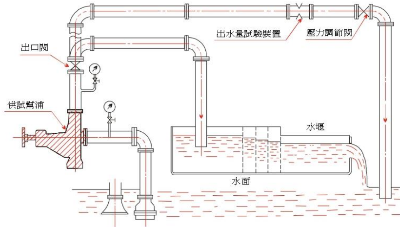
附圖2 試驗裝置示意圖
