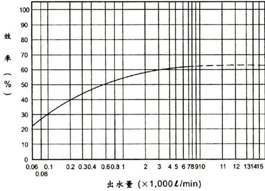
附圖3 幫浦效率曲線
