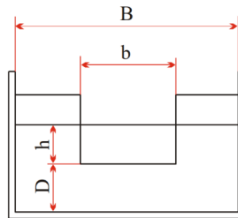
圖11 四角堰
