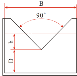
圖10 直角三角堰
