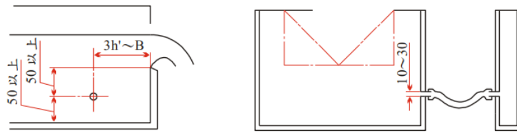
圖8 堰水頭之測定位置 (單位：mm)
