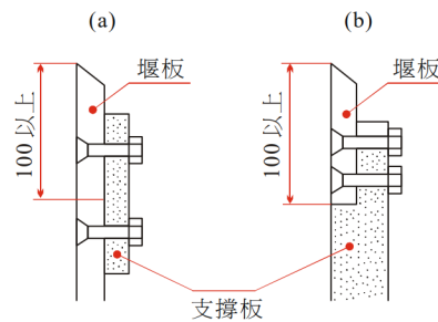
圖2 堰板之內面圖 (單位：mm)
