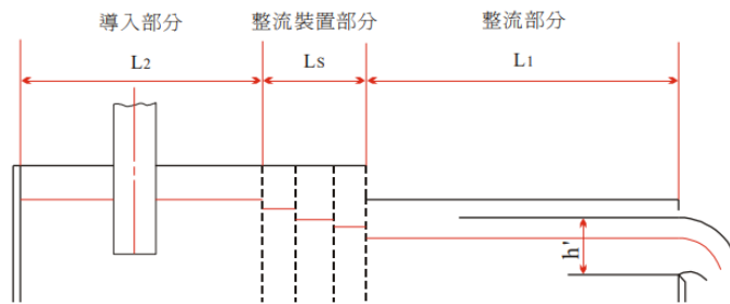
圖6 水路
