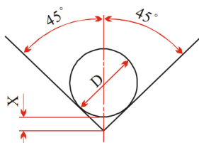
圖9 三角堰水頭零點之測定
