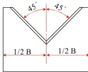
圖3 直角三角堰之切口
