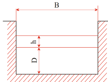
圖 12 全幅堰
