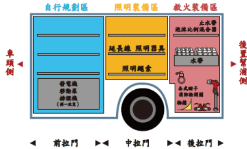
消防機關消防車輛搶救器材擺放位置一致化示意圖 適用車種：水箱消防車
