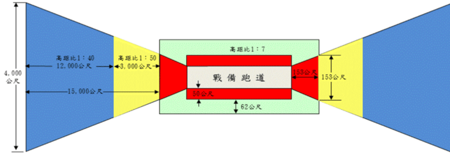
機場戰備跑道禁、限建範圍示意圖
