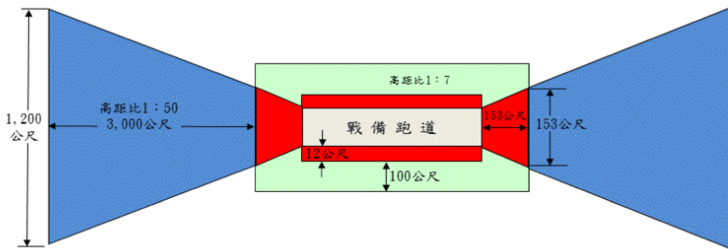
公路戰備跑道禁、限建範圍示意圖
