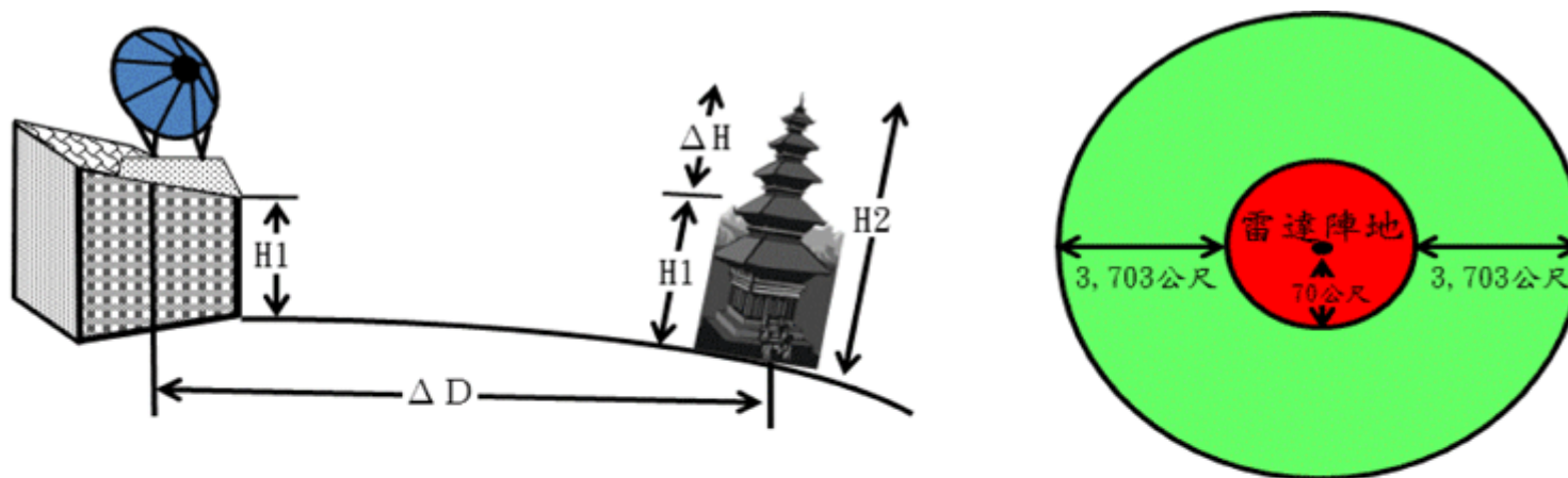
戰管雷達陣地禁、限建範圍示意圖
