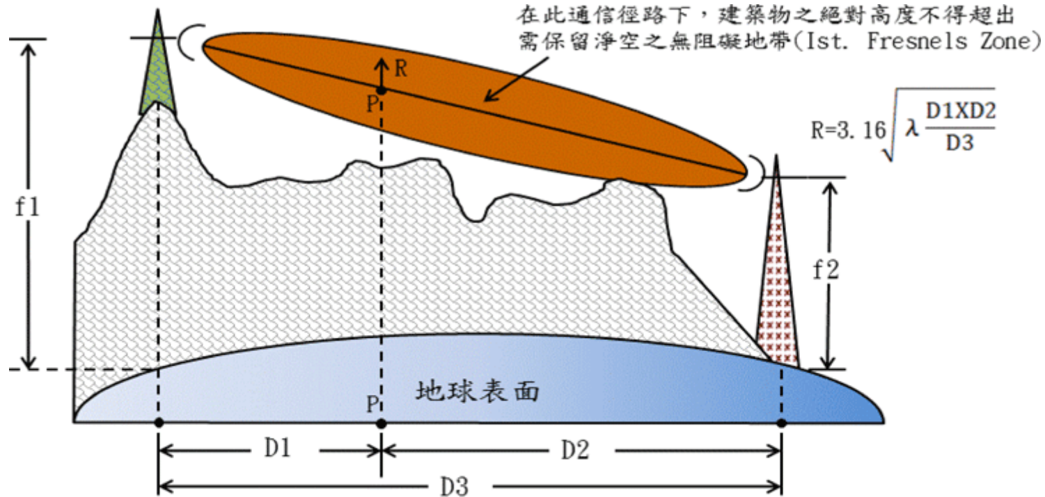
衛星及微波通信放射電波管制區限建範圍、高度示意圖
