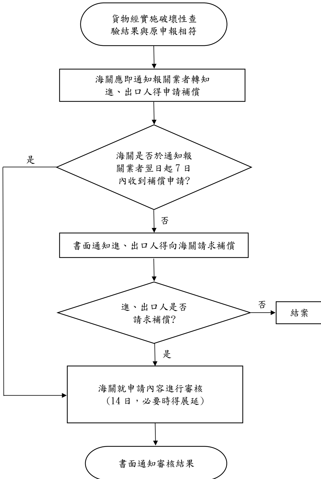
海關實施進出口貨物破壞性查驗補償處理程序流程圖
