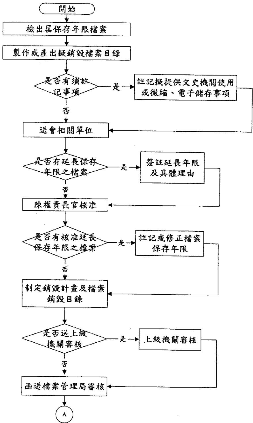
圖 17-1 屆保存年限檔案銷毀作業流程
