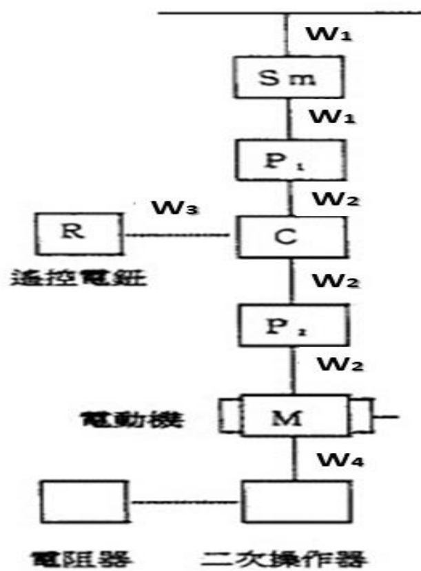
圖一五三 標準電動機分路圖
