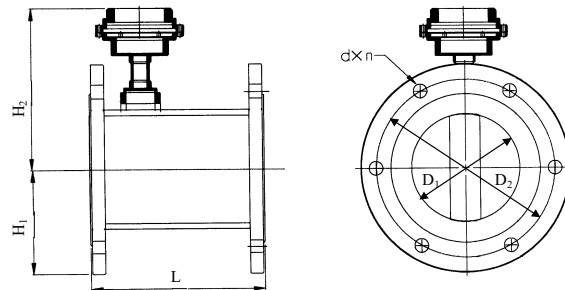
圖 C.1 渦流型水量計凸緣尺度
