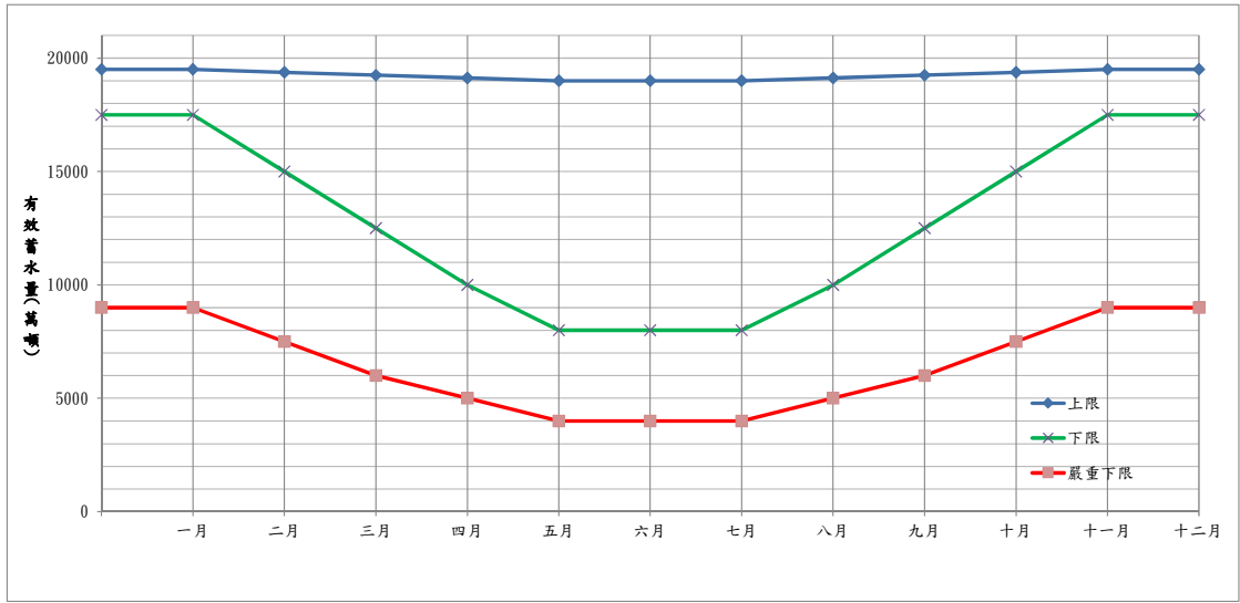
附圖 石門水庫運用規線圖
