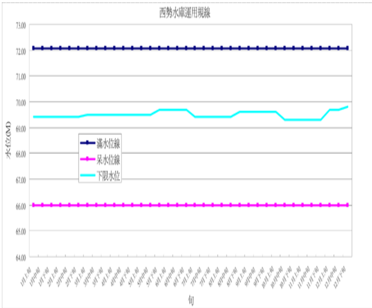
西勢水庫運用規線圖
