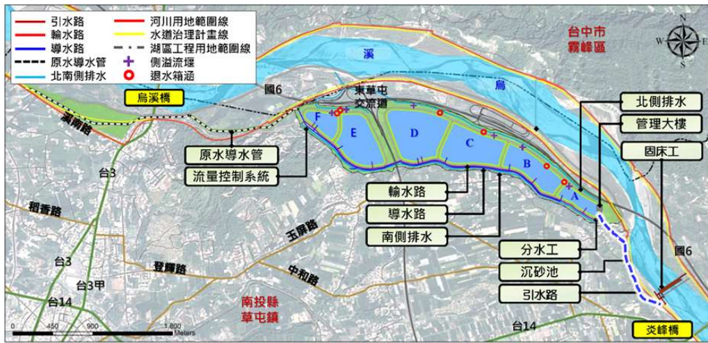
附圖一 烏嘴潭人工湖設施位置圖
