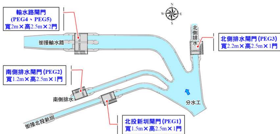
附圖三 人工湖區各設施閘門位置圖
