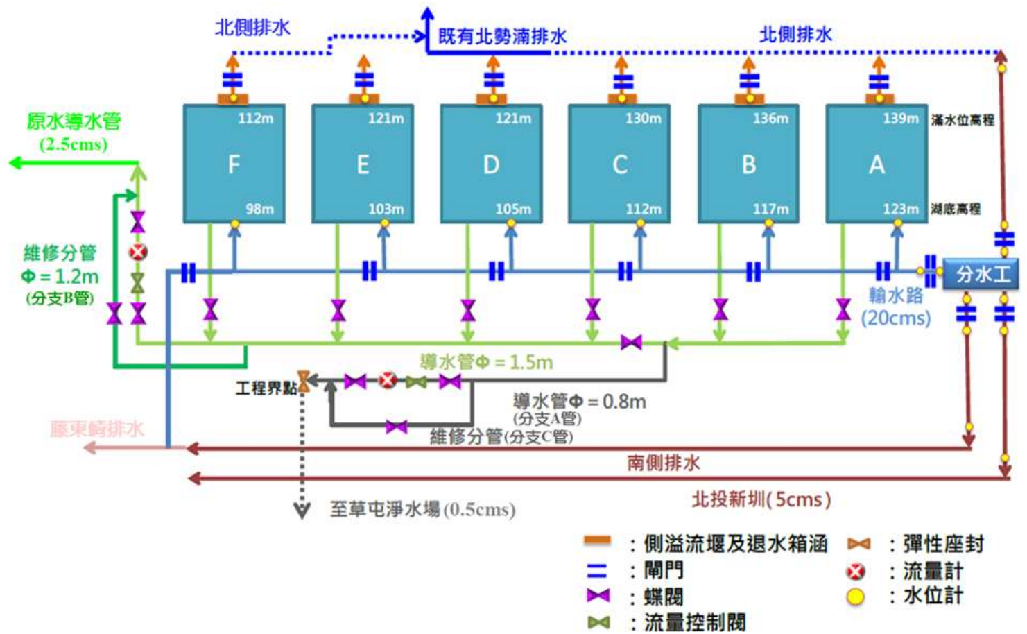
附圖四 人工湖區供水系統簡圖
