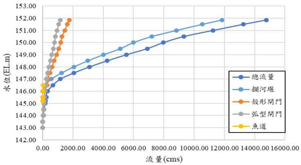
附圖五 固床工之流量率定曲線圖
