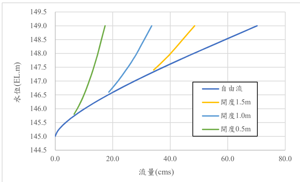
附圖六 取水口開門(開啟一門)水位-開度-流量圖
