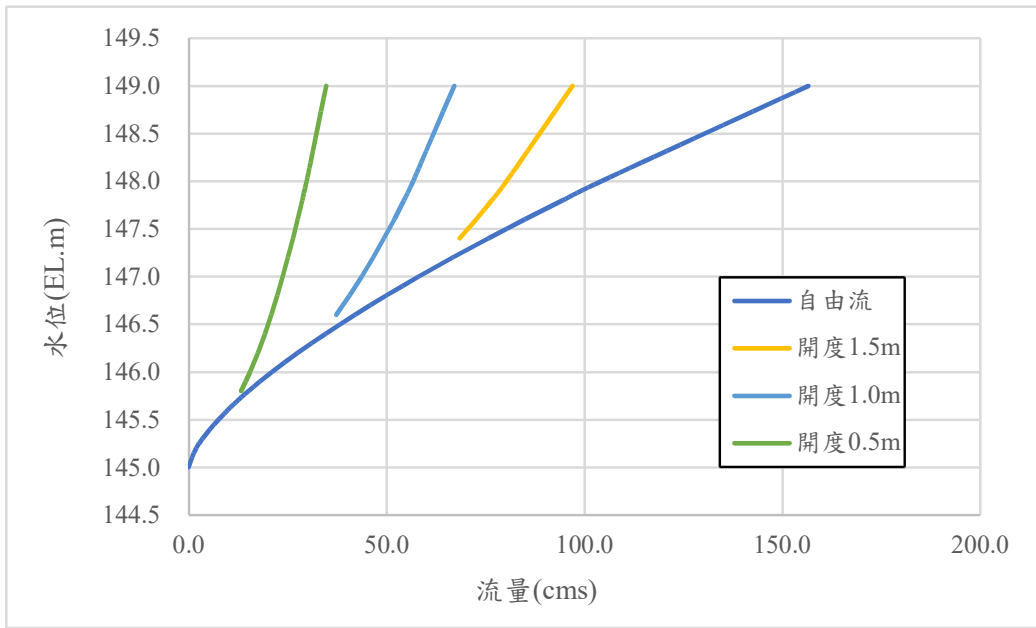
附圖七 取水口閘門(開啟二門)水位-開度-流量圖
