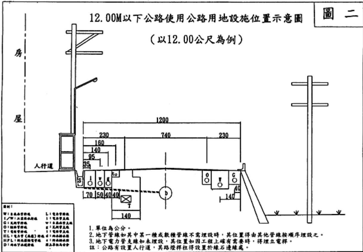
12.00M以下公路使用公路用地設施位置示意圖
