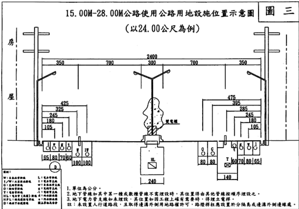
15.00M-28.00M公路使用公路用地設施位置示意圖
