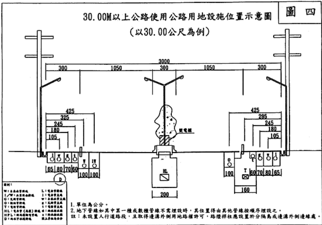
30.00M以上公路使用公路用地設施位置示意圖
