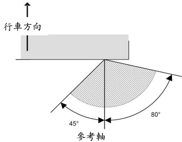
圖二：尾燈(適用4.6.1之 M/N/O/L 類車輛及4.6.2.2之 L 類車輛)
