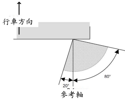
圖二之一：安裝後車輛尾燈之 H 平面距地高不超過七五〇公釐者角度(適用4.6.1之 M/N/O/L 類車輛)
