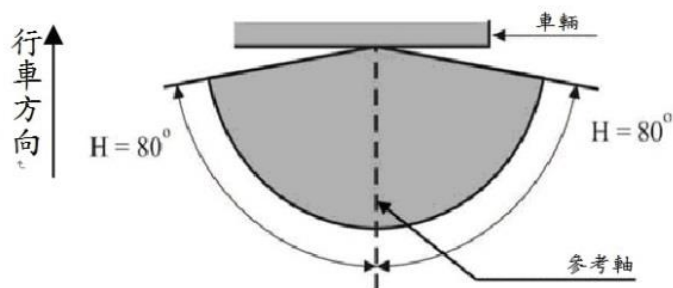
圖三：適用4.6.2.1之 L 類車輛單燈式尾燈水平照射角度
