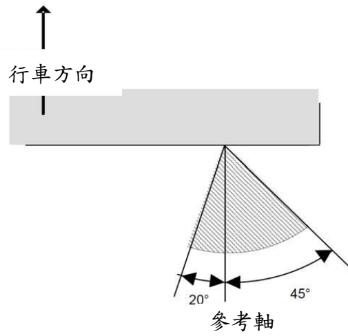
圖二之一：安裝後煞車燈(S1及S2)之H平面距地高不超過七五〇公釐者(適用4.4.1之M/N/O/L類車輛)
