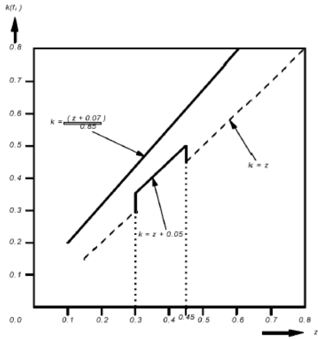
圖一 A M_1 及特定N1類車輛
