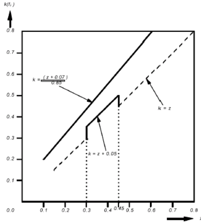
圖一A：6.6.1.2.1 所述 N1 類車輛
