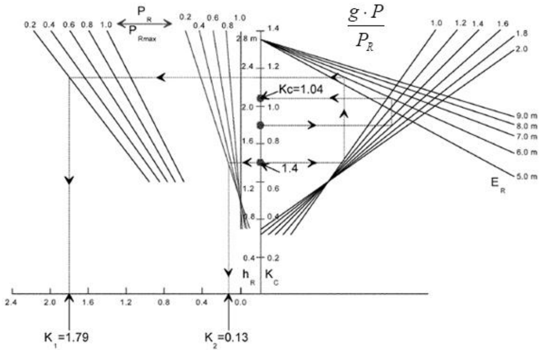
圖四 B (參見本法規6.3.3與圖四 A)
