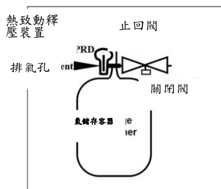
圖一、典型壓縮氫儲存系統
