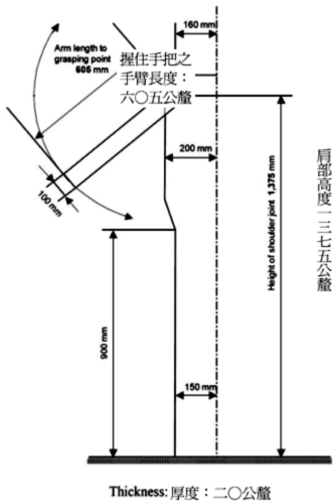
圖五 手把測量裝置
