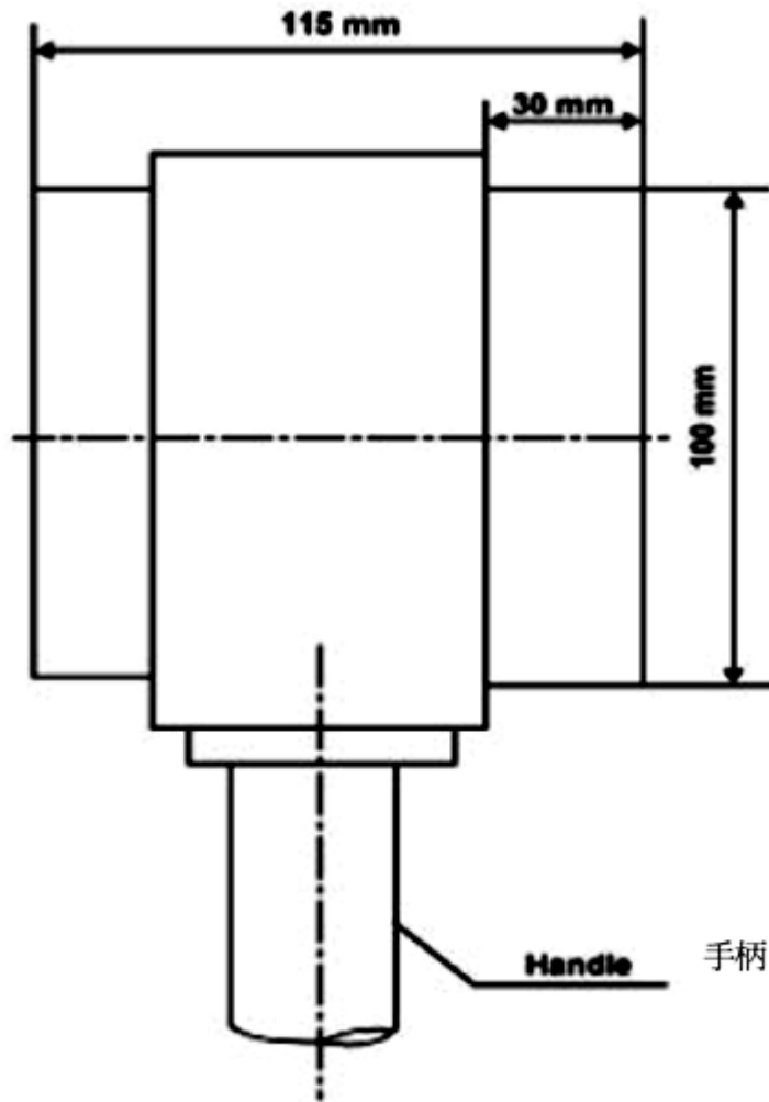
圖七 車門關閉力測量裝置
