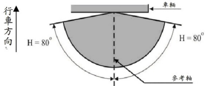
圖二之一：安裝後車輛尾燈之 H 平面距地高不超過七五〇公釐者角度(適用 4.6.1 之 M/N/O/L 類車輛)
